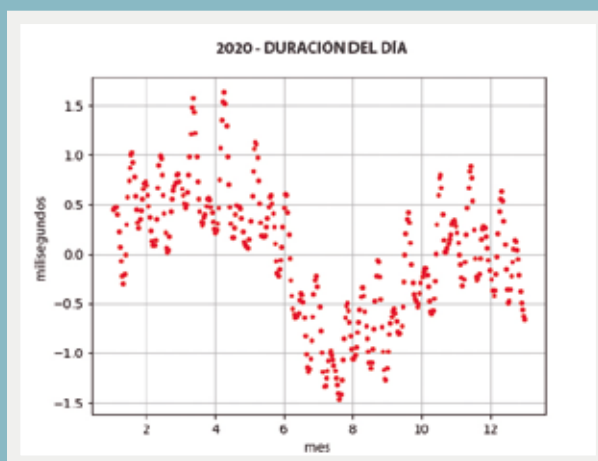
Figura 2. Duración del día durante el año 2020, en su exceso respecto a 86400 segundos. Se advierten los periodos de anual y semestral de variación de la velocidad de rotación y una aceleración durante el año 2020. Ya fue anunciado que no será necesario intercalar 1 segundo a fines del 2021. (Fuente de datos: Serie C04 de parámetros de orientación terrestre del IERS).
